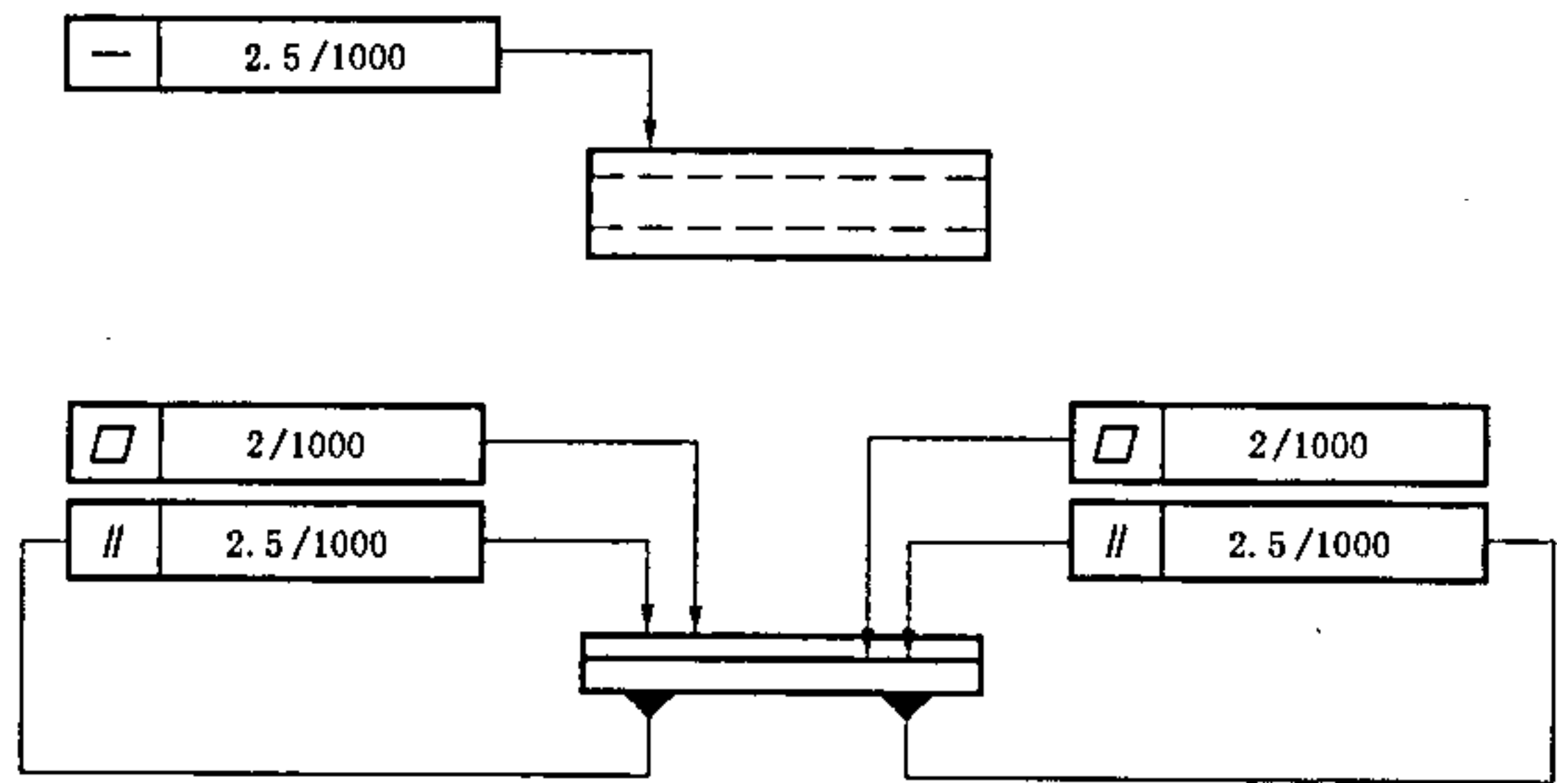
图 A.10 形位公差
