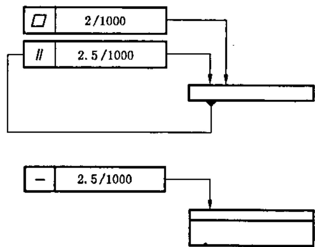
图 A.8 形位公差
