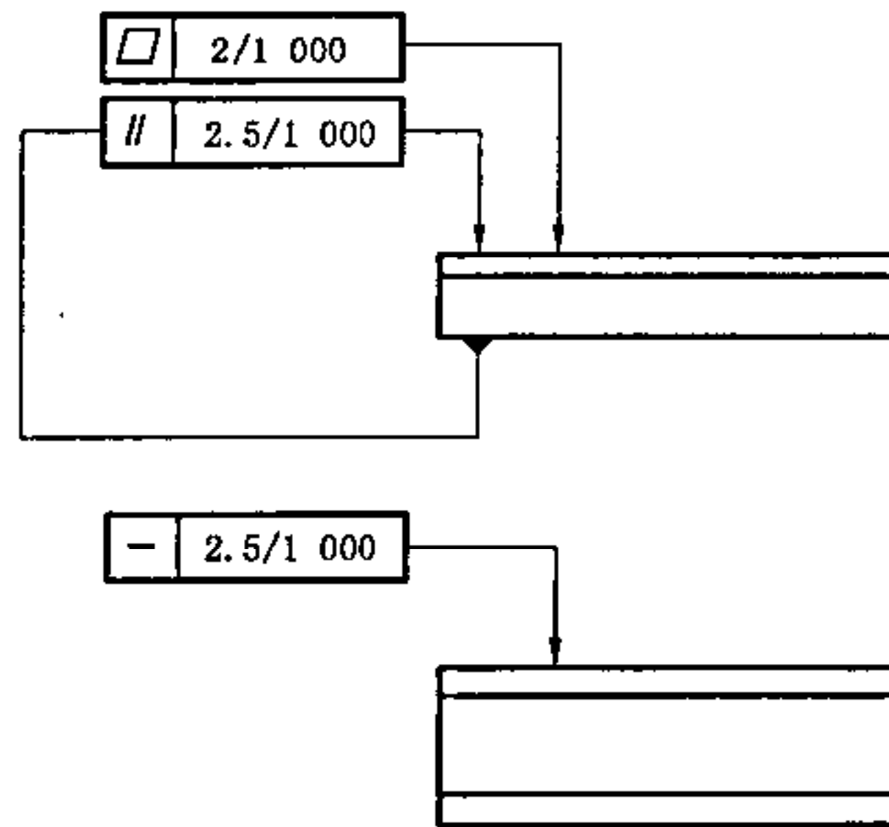
图 A.2 形位公差
