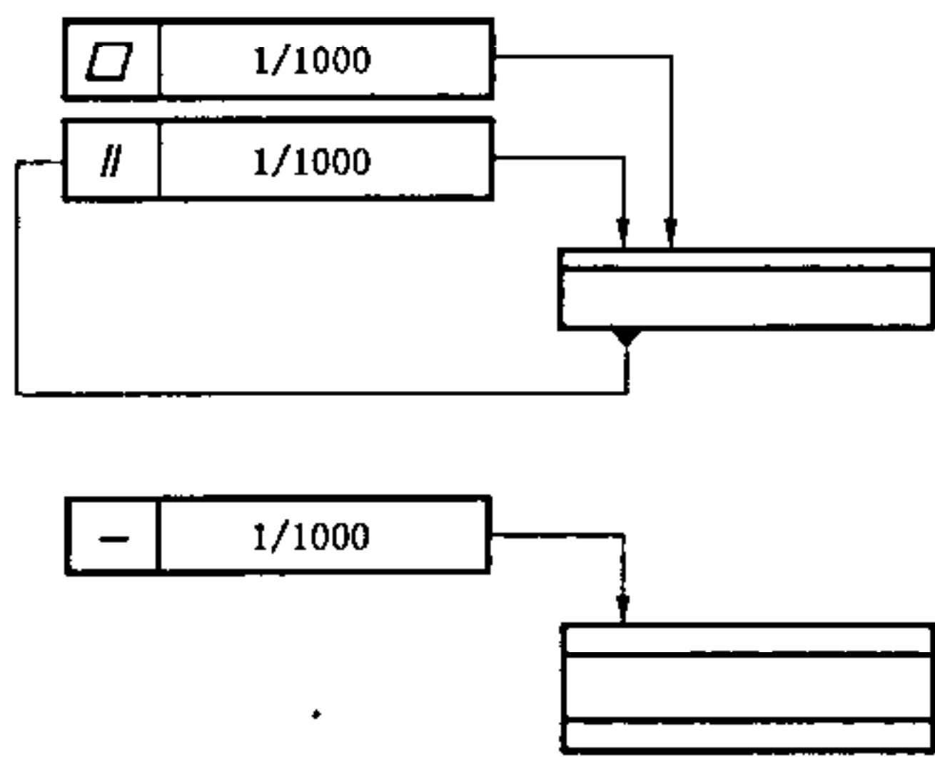
图 A.6 形位公差
