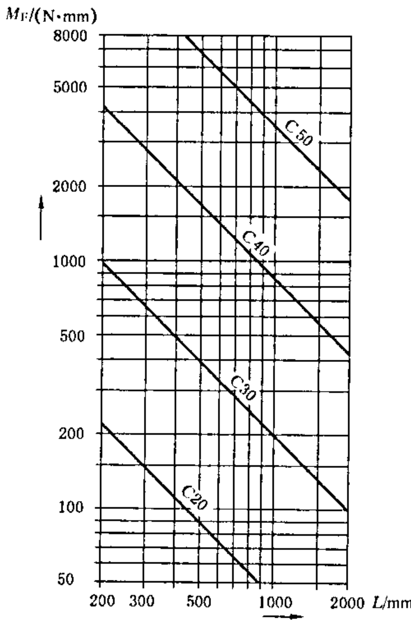
图 B.5 允许负载能力 M_E = f(L)
