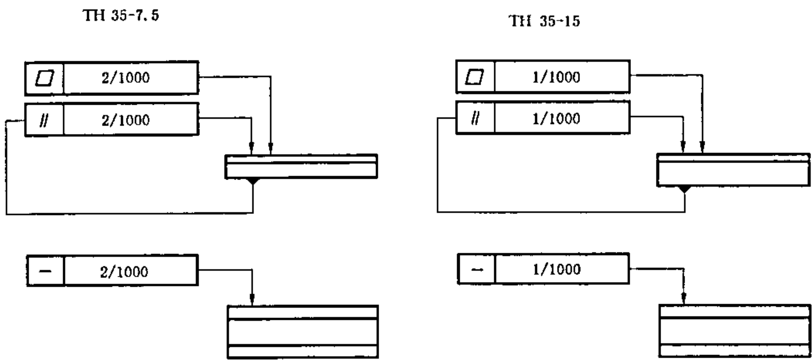
图 A.4 形位公差
