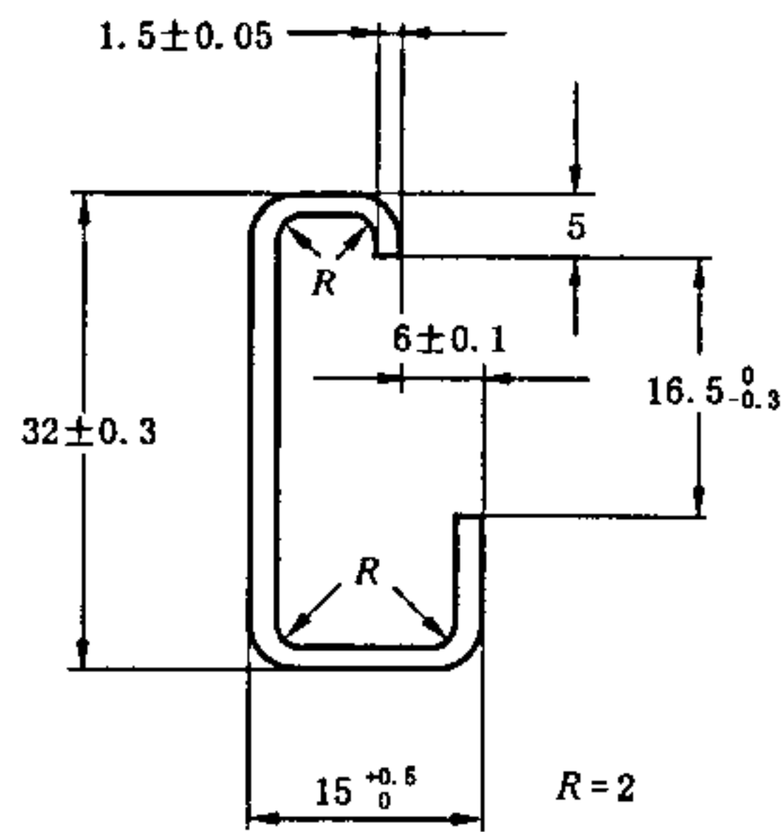
图 A.9 “G”型轨(尺寸单位:mm)
