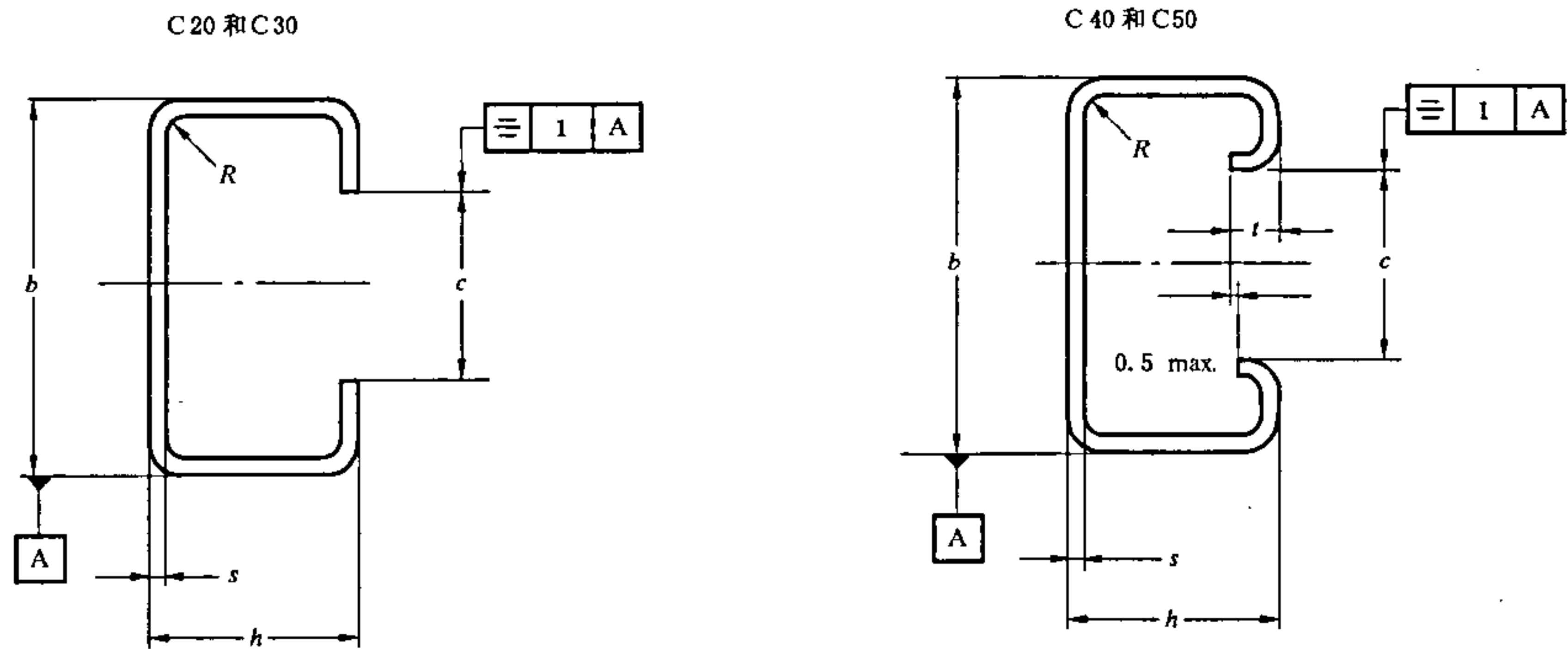
图 A.7 “C”型轨
