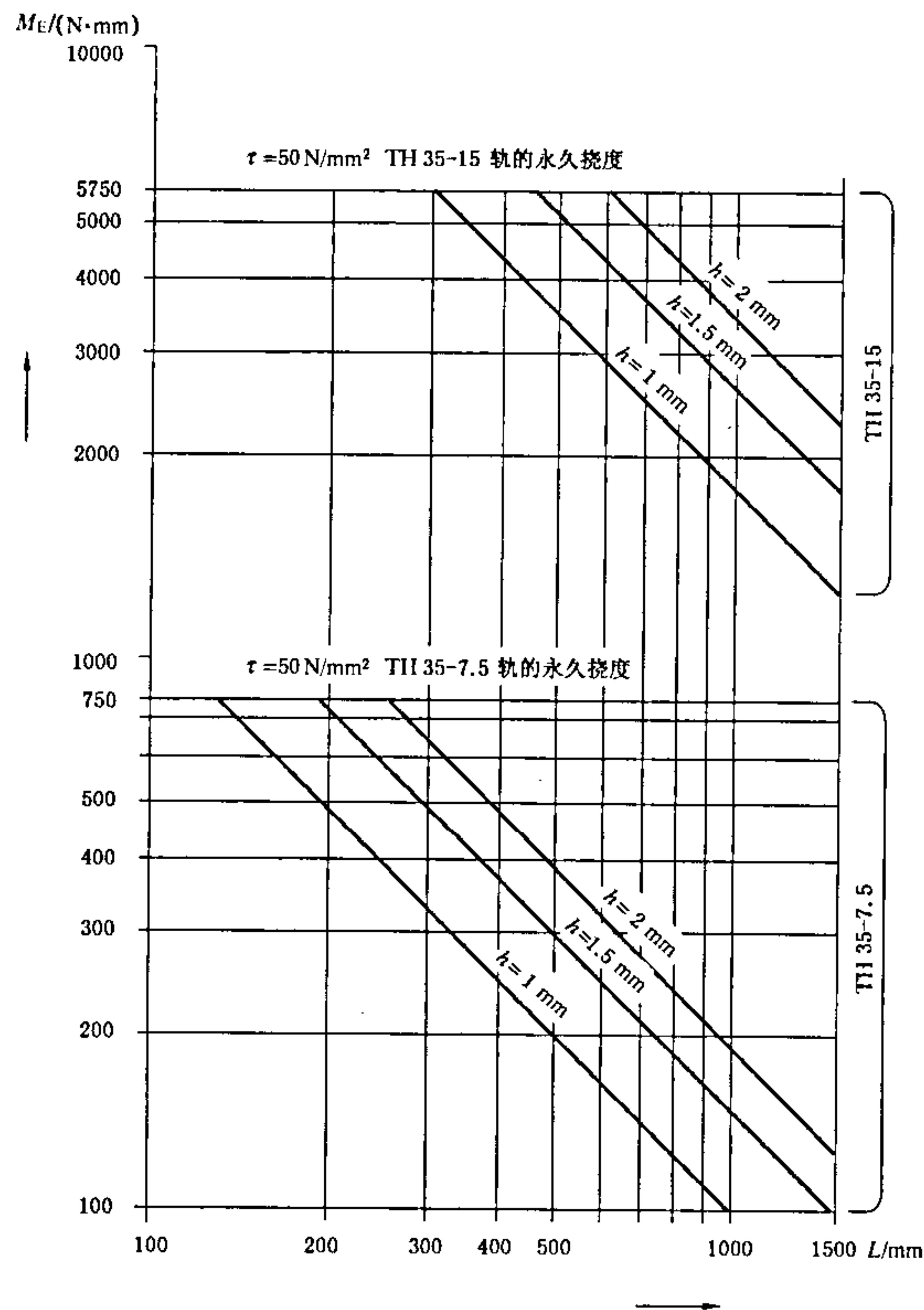
图 B.2 允许负载能力 M_E = f(L, h)
