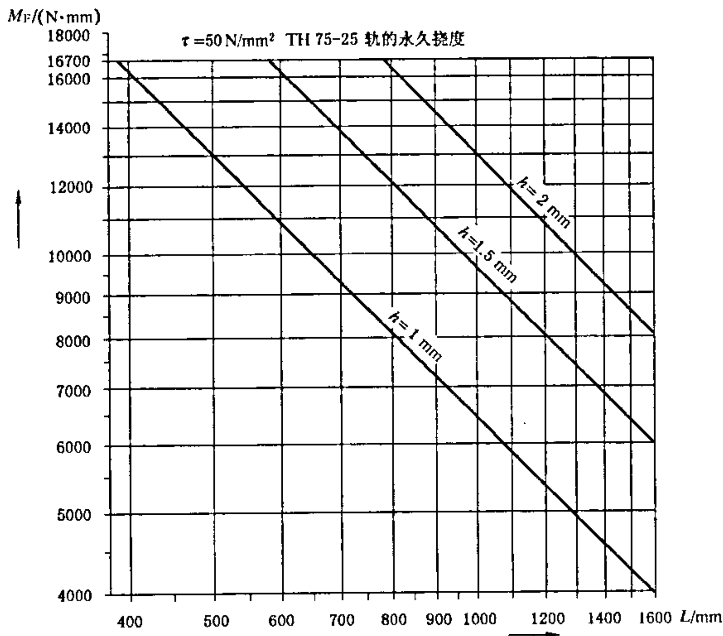
图 B.3 允许负载能力 M_E = f(L, h)
