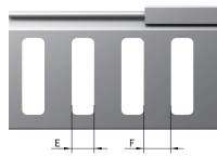
Slot 出线孔示意图
