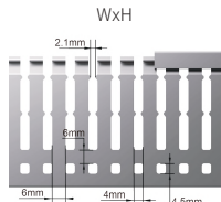
Narrow Slot (SR) 出线孔示意图
